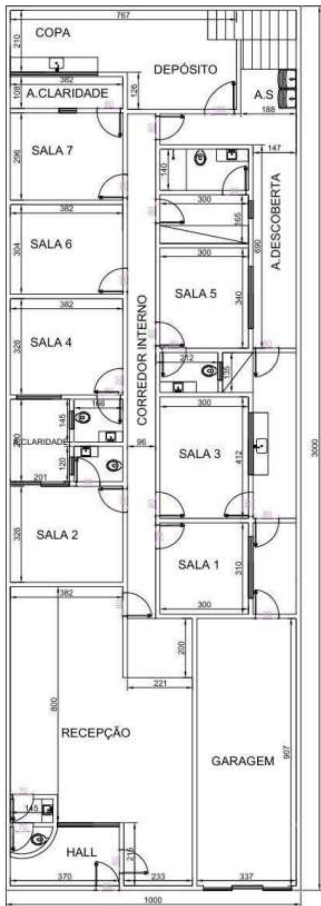
PLANTA BAIXA - ANDAR TÉRREO
