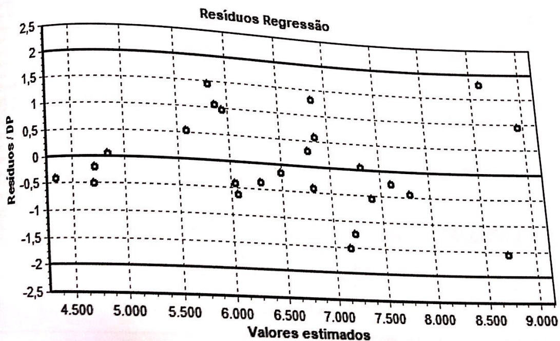
Gráfico de resíduos - Regressão Linear
