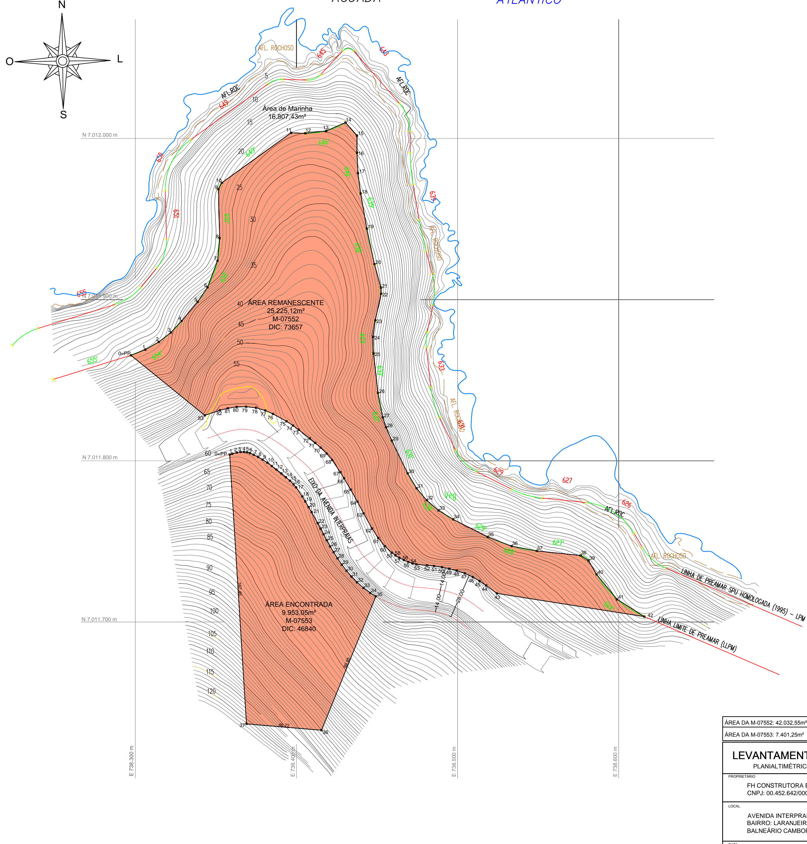
PLANTA CONFORME ÁREA ENCONTRADA
