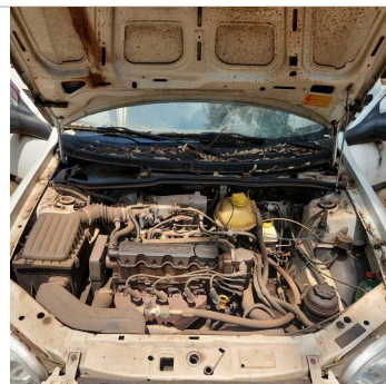
MOTOR COMPARTIMENTO
