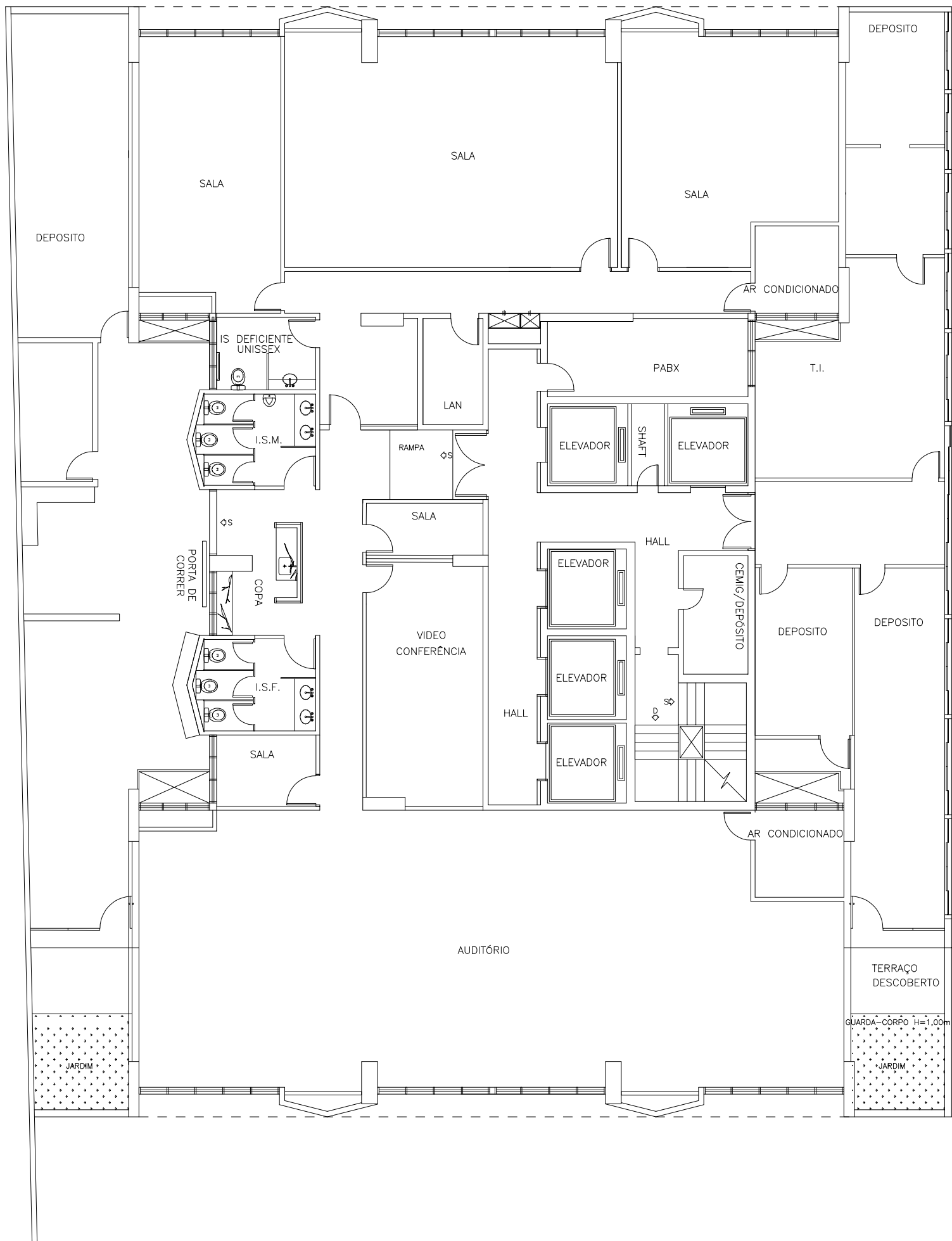
PLANTA PILOTIS
